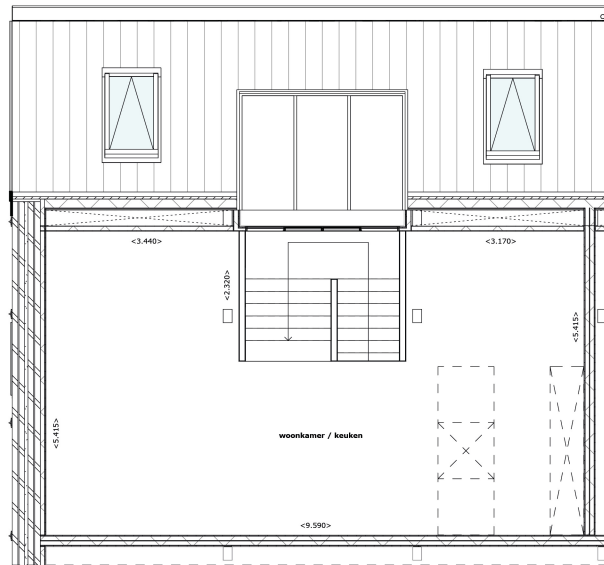
Plattegrond verdieping 04 1:50
